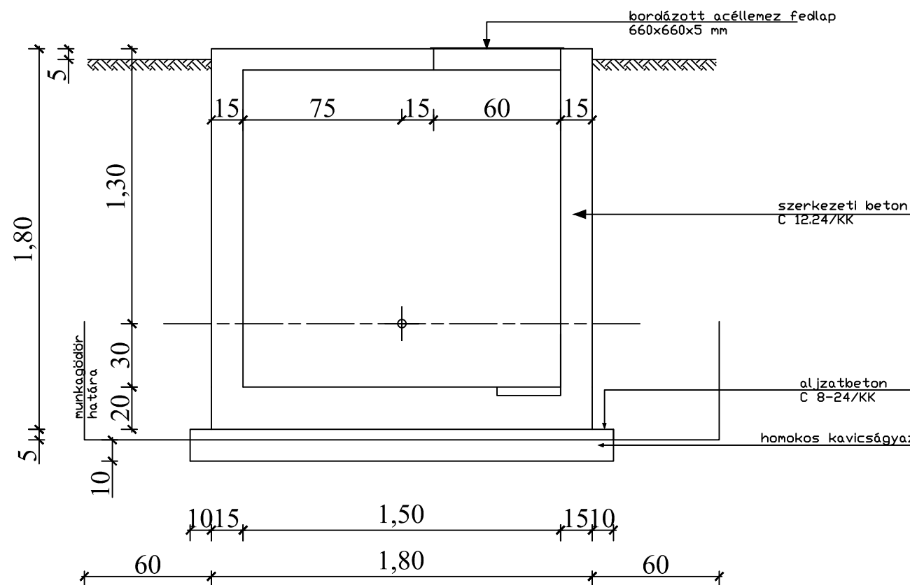
A-A METSZET
