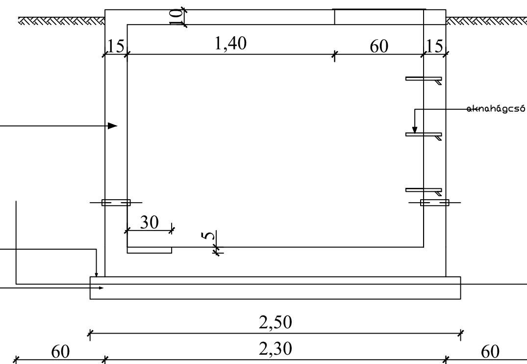
B-B METSZET
