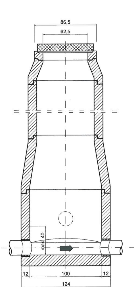
B-B metszet
