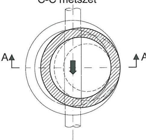
C-C metszet
