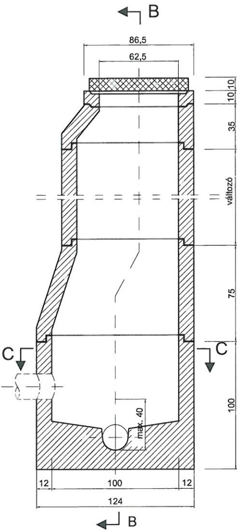
A-A metszet
