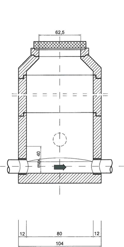
B-B metszet
