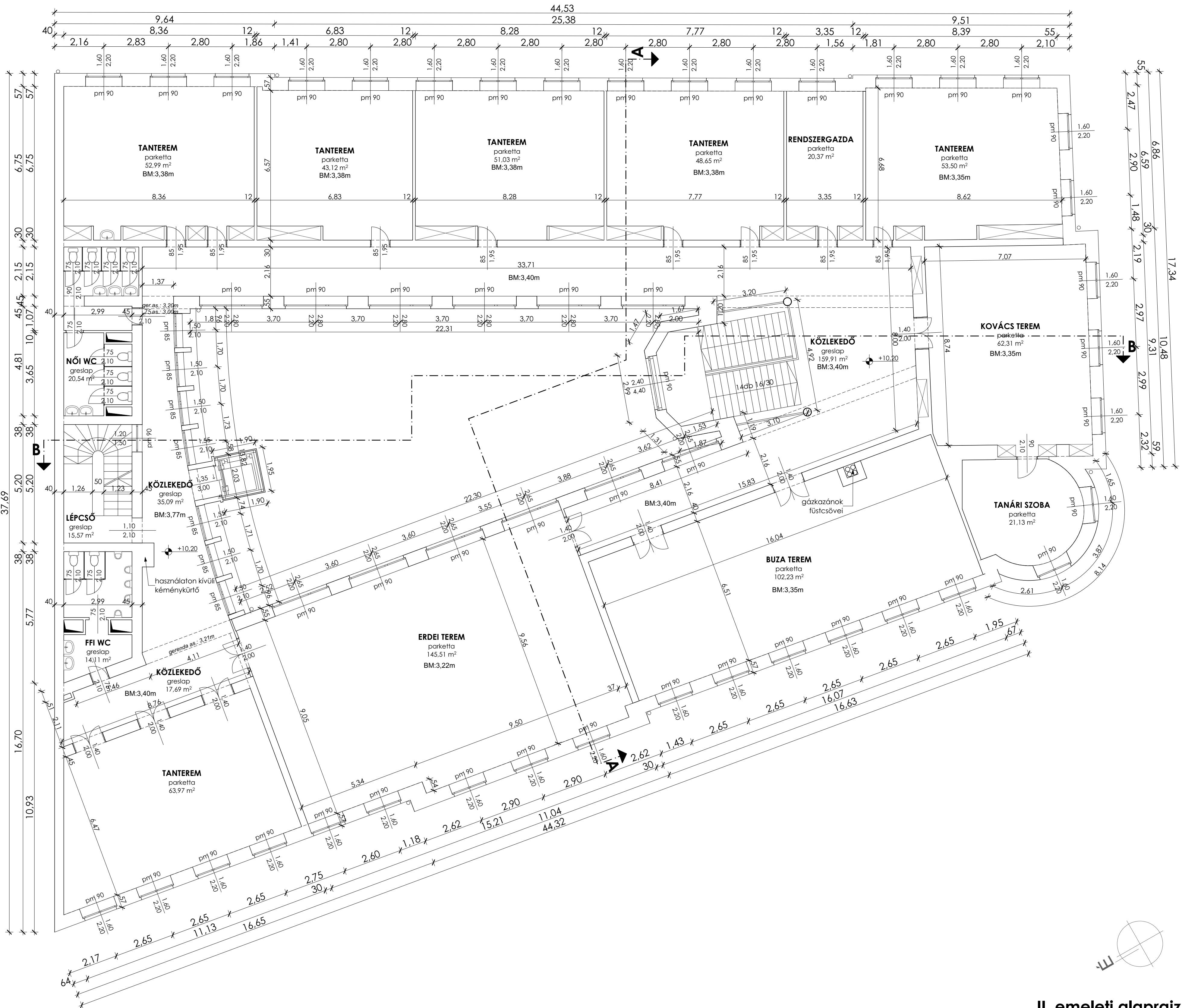
II. emeleti alaprajz m=1:100
